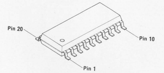
TC74HC244AF (Q1010, 1016)
