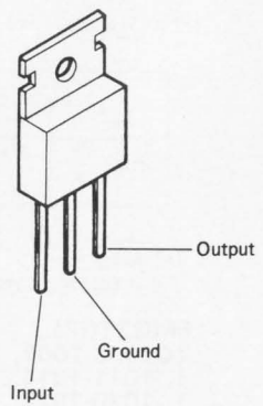
HA17805P (Q1001)
