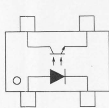
TLP181 (Q1023)
