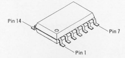
MC74HC00FL (Q1019)
