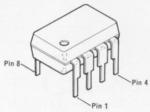
BR93C56 (Q1002)
