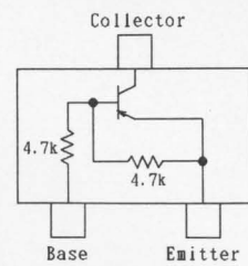
DTA143XK (Q1024)
